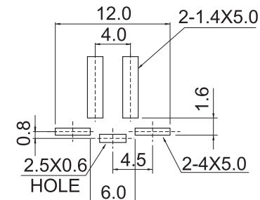
P.C.B.Land Pattern
