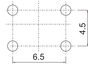
P.C.B.Land Pattern
