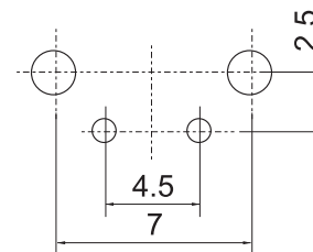
P.C.B.Land Pattern
