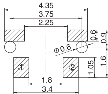
安装参考图
