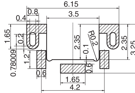
安装参考图
