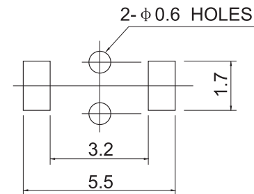
P.C.B.Land Pattern
