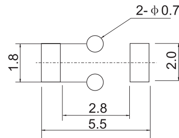
P.C.B.Land Pattern
