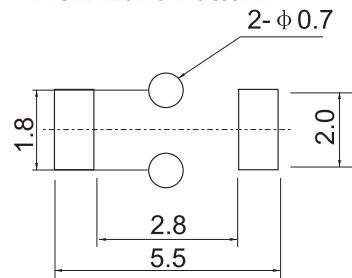
P.C.B.Land Pattern
