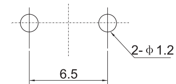
P.C.B.Land Pattern
