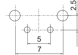
P.CB.Land pattern
