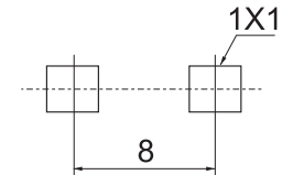
P.C.B.Land Pattern
