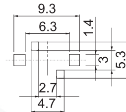
P.C.B.Land Pattern
