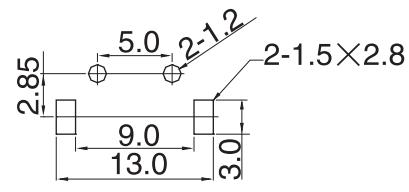
P.C.B.Land Pattern
