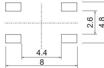
P.C.B.Land Pattern
