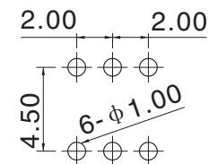
PCB Layout(Pattern Side)
