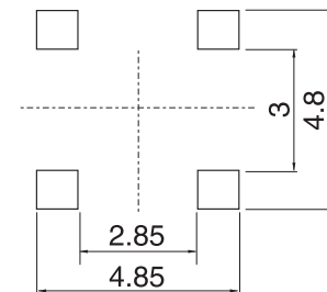
P.C.B.Land Pattern
