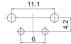
P.C.B. Land Pattern
