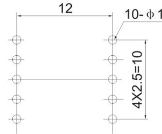
P.C.B.Land Pattern
