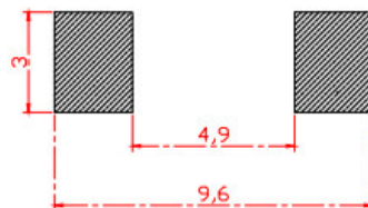
PCB. 焊接图
